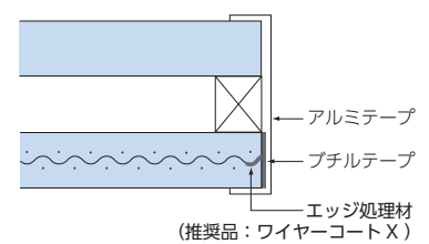
【複層ガラス】
