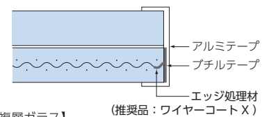
【複層ガラス】
