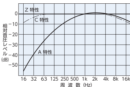
騒音計のA、C、Z特性
