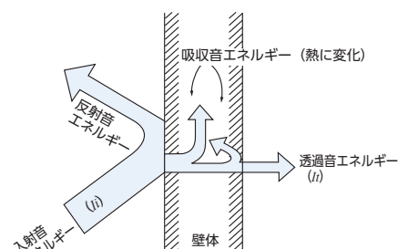
音のエネルギー経路
