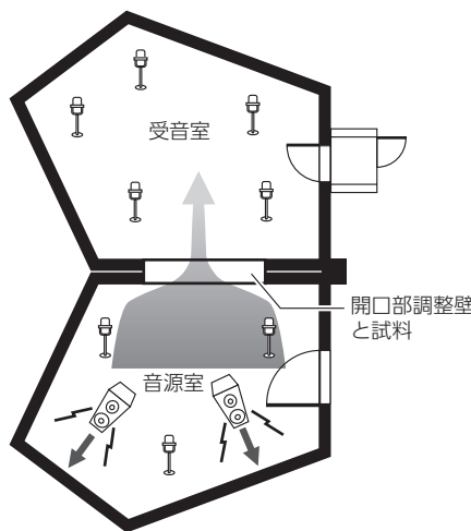
【図1】タイプⅠ試験室
