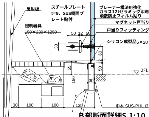
B部断面詳細S.1:10
