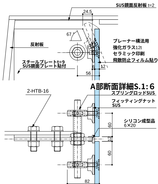
A部断面詳細S.1:6
