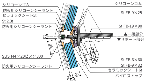
縦材横断面図 S.1:5
