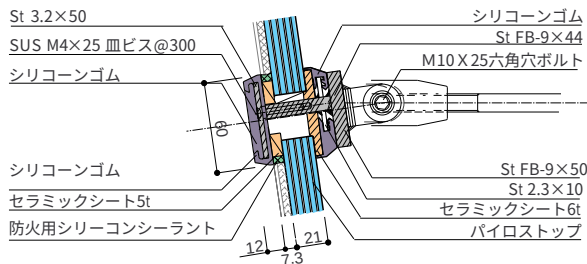
横材縦断面図 S.1:5
