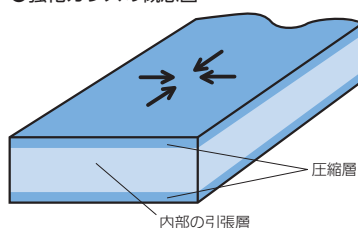
●強化ガラスの概念図
