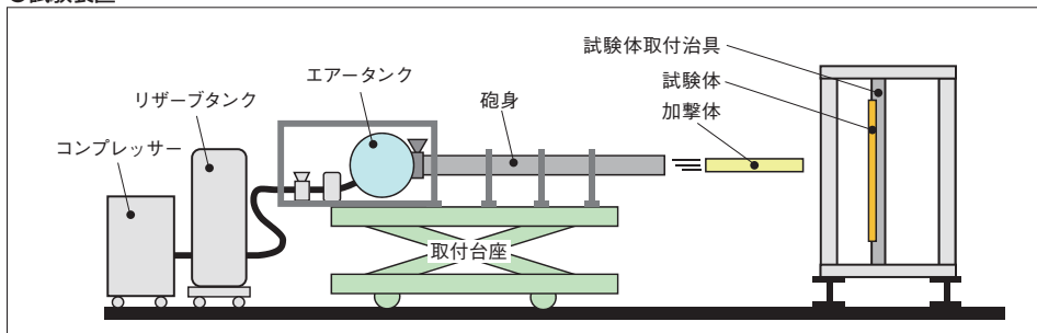
加撃体B~E:木片
