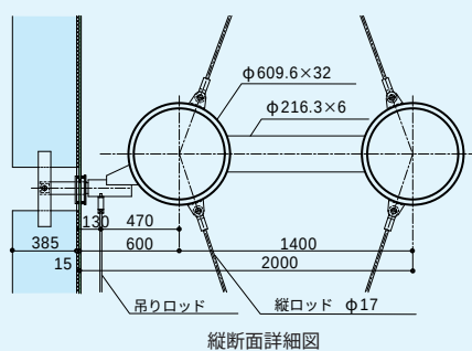
縦断面詳細図
