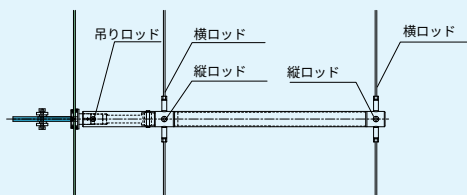
平面詳細図
