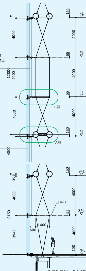
全体矩形図 S.1.200
