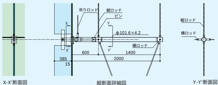
X-X'断面图
