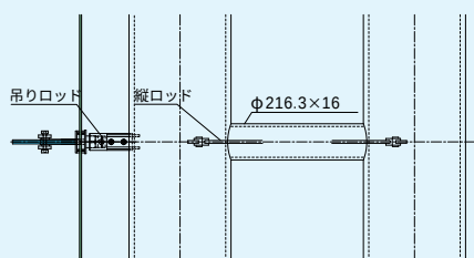
平面詳細図
