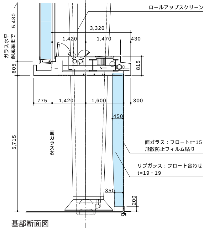
アトリウムエントランス・カーテンウォール詳細図 S.1 : 100
