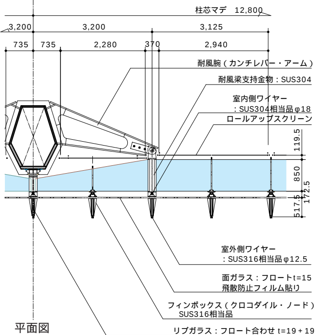
アトリウムエントランス・カーテンウォール詳細図 S.1 : 100
