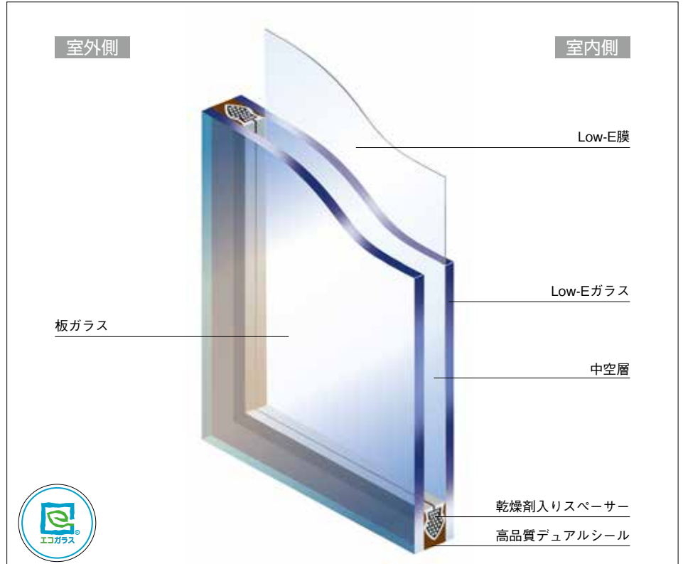
ペアマルチスーパー構造図
