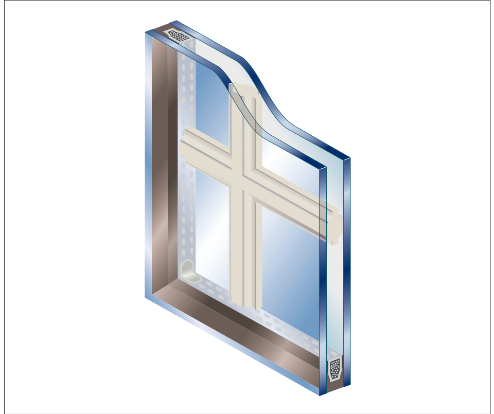
ペアマルチクロス構造図
