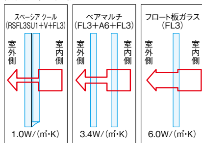
熱貫流率の比較
