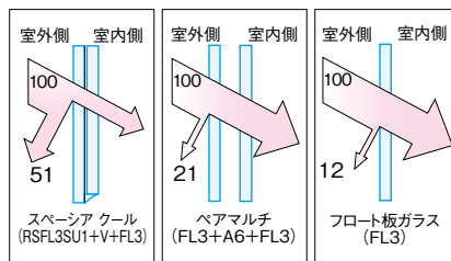
日射熱除去率の比較
