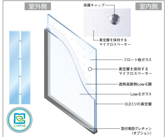
スペーシア クール構造図
