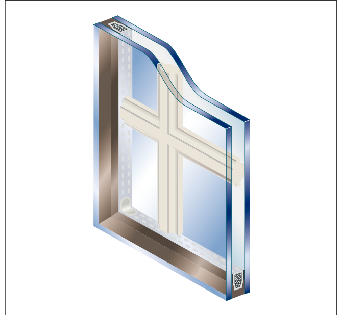
ペアマルチクロス構造図
