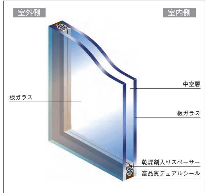
ペアマルチ構造図
