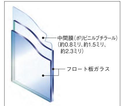
セキオ30、60、90構造図
