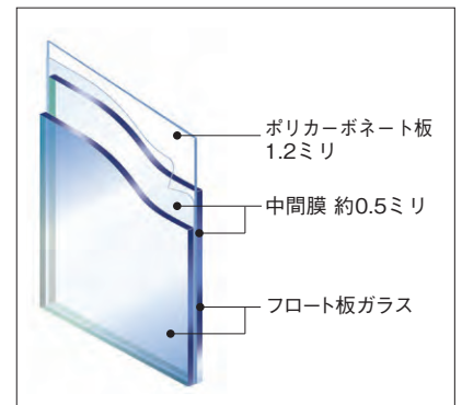
セキオSP構造図
