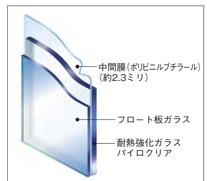
セキオPY構造図
