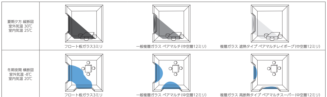
【図】平均放射温度分布 室内断面図(部屋寸法/2.7×2.7×2.7m 窓寸法/1.35×1.35m 腰壁/0.9m 窓配置/南面および西面)
