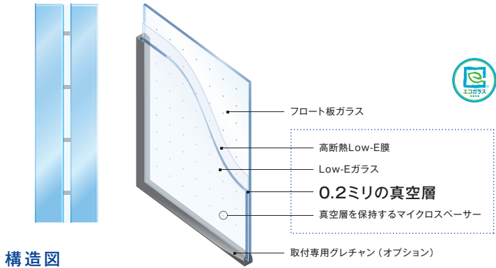
構造図
