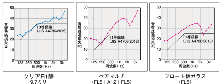
遮音性能の比較
