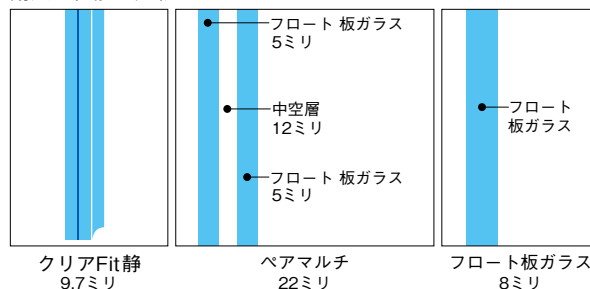
耐風圧性能の比較
