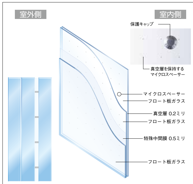
クリアFit静 構造図
