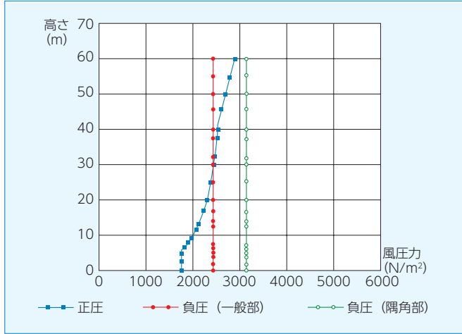
【図3】風圧力とガラスの地上高さの関係(建物基準高さと軒高さの平均が60mで再現期間100年の場合)粗度区分Ⅲ、風速34m/s
