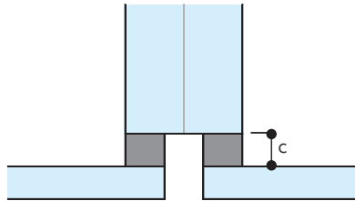
【図4】構造シーラントの接着厚
