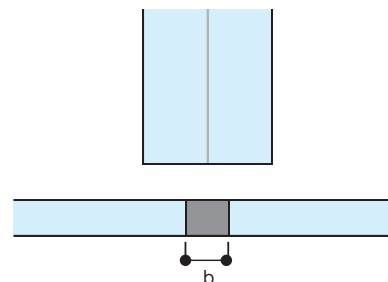
【図3】面ガラス間のクリアランス
