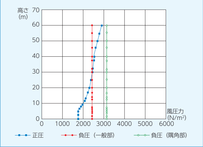
【図3】風圧力とガラスの地上高さの関係(建物基準高さと軒高との平均が60mで再現期間100年の場合)粗度区分Ⅲ、風速34m/s
