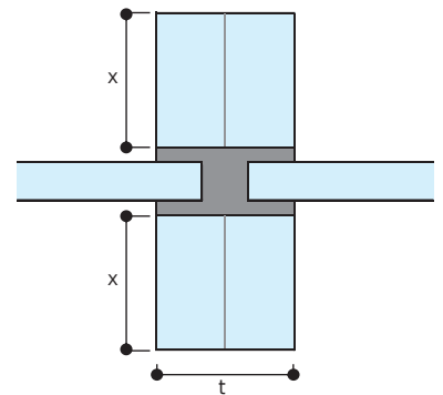
【図7】両側方立タイプ
