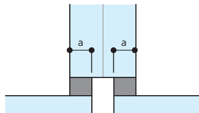
【図1】構造シーラントの接着幅
