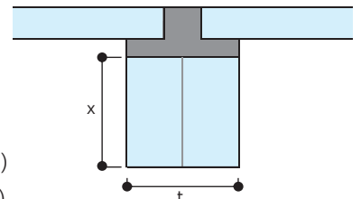
【図8】片側方立タイプ
