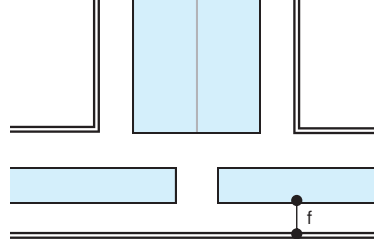
【図5】面ガラス間のクリアランス
