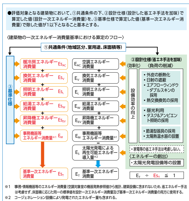
【図1】建築物の一次エネルギー消費量基準の考え方
