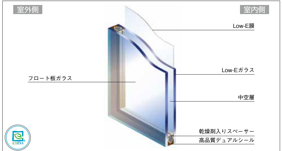
ペアマルチEA寒冷地タイプ構造図
