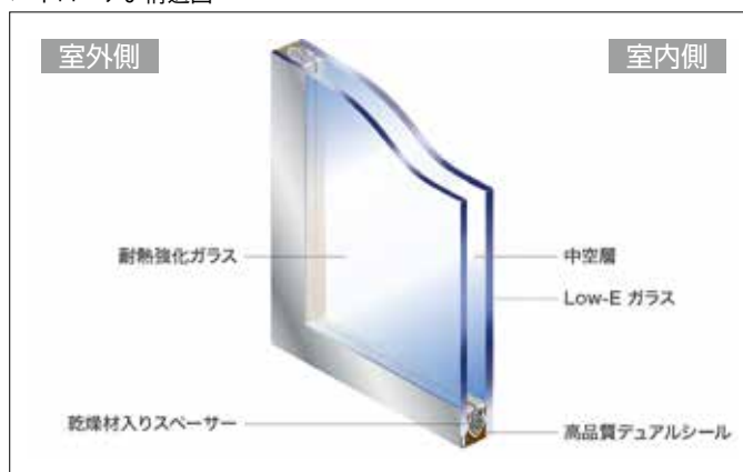
パイロペアJ 構造図
